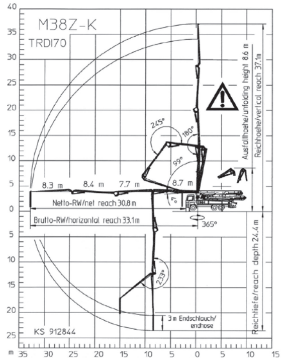
Betonpumpe Reno II Typ Putzmeister BFS 38-4 mit 38 m Verteilmast 4-Achs, 32 t
